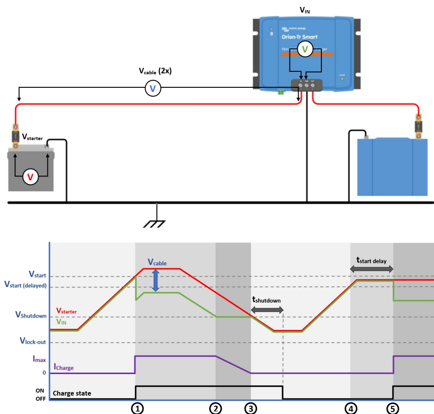
Afbeelding 8: Werking motoruitschakelingsdetectie
