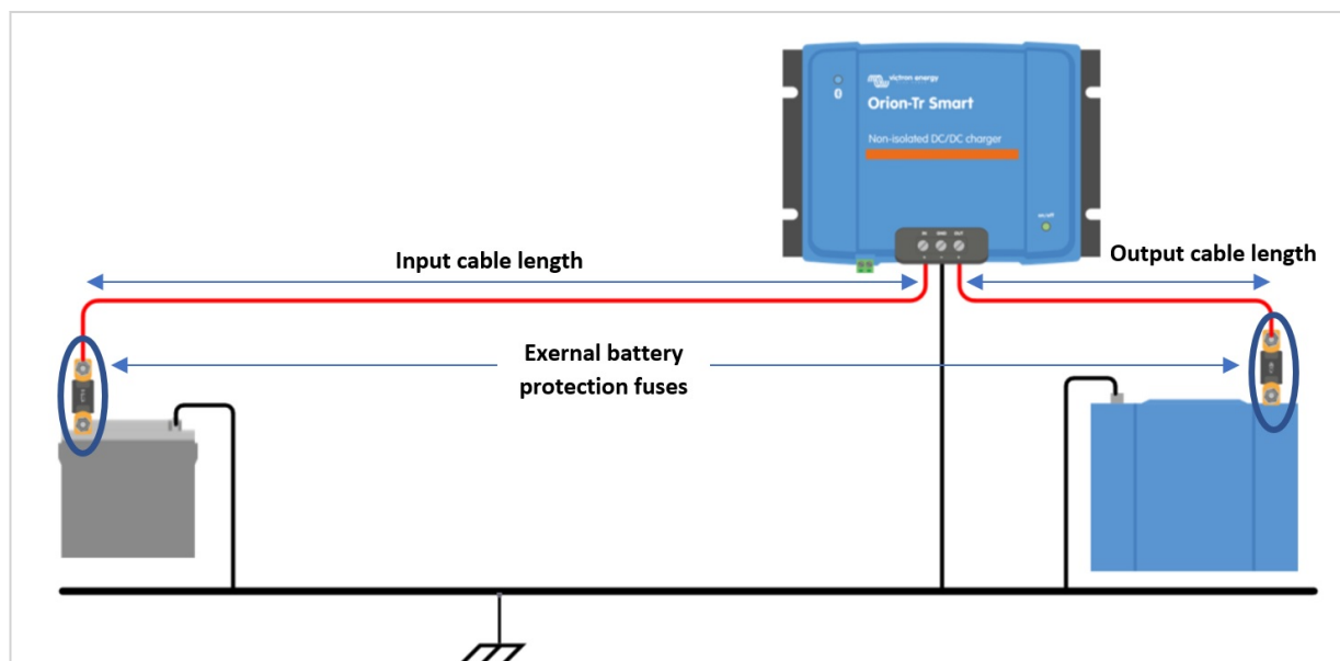
Afbeelding 6: Aanbevelingen voor kabels en zekeringen
